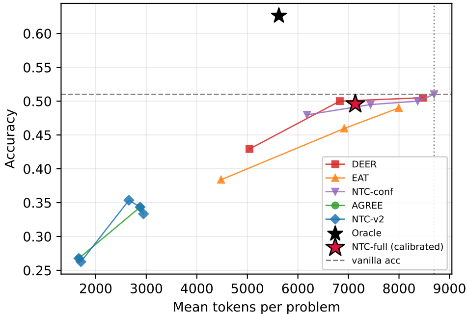
Qwen3-4B · gpqa_diamond (n=198)
