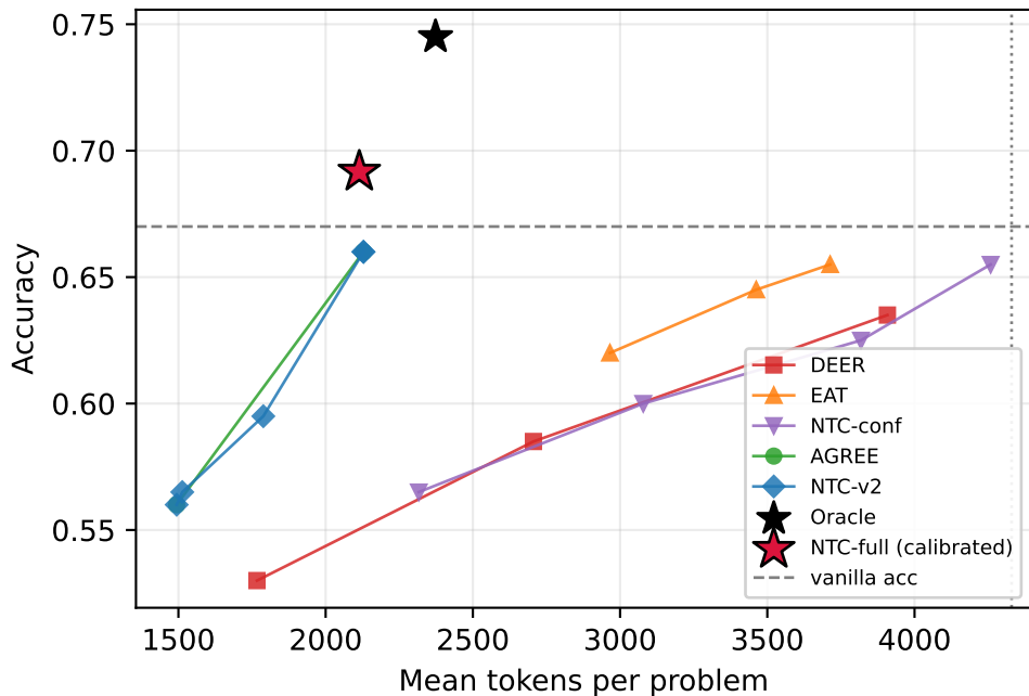
Qwen3-4B · math500 (n=200)
