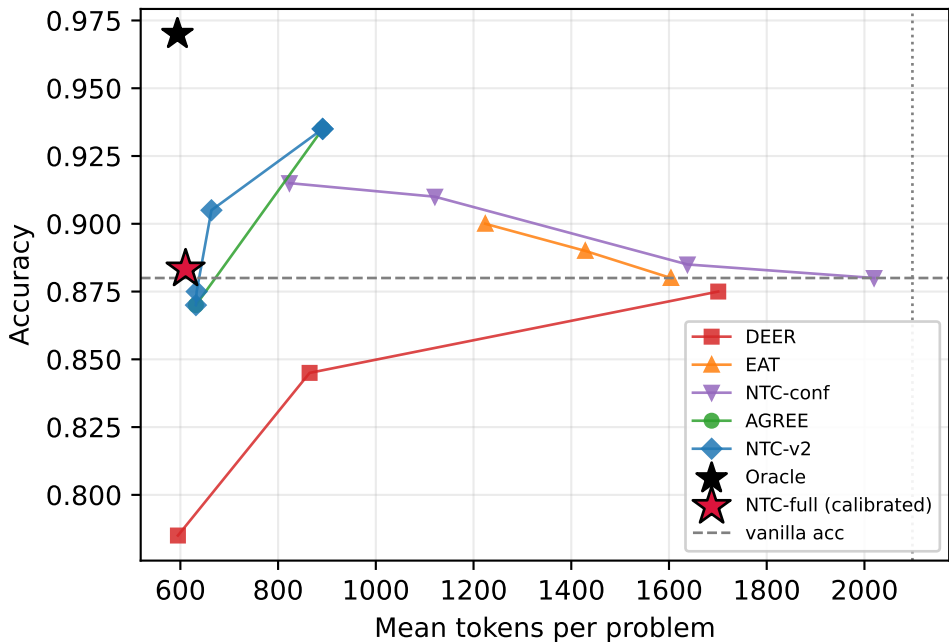
Qwen3-4B · gsm8k (n=200)
