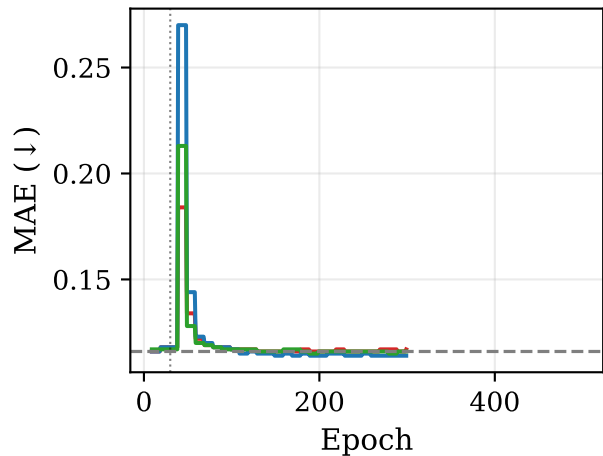
CN15K: MAE ( \downarrow )
