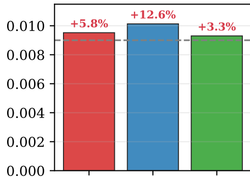
CN15k: MSE ( \downarrow )
