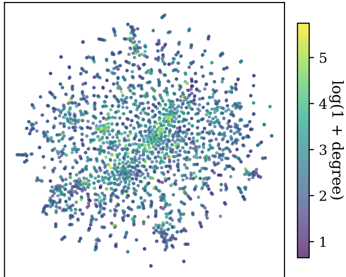
CN15K — Spectral init
