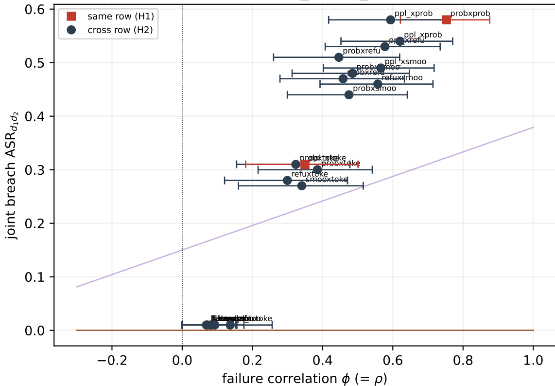
Figure 3(a): hpc_vicuna_autodan
