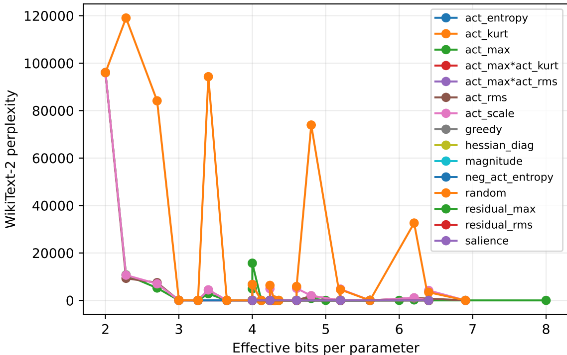
meta-llama/Llama-3.2-1B
