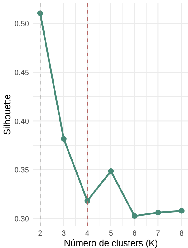
Silhouette promedio
