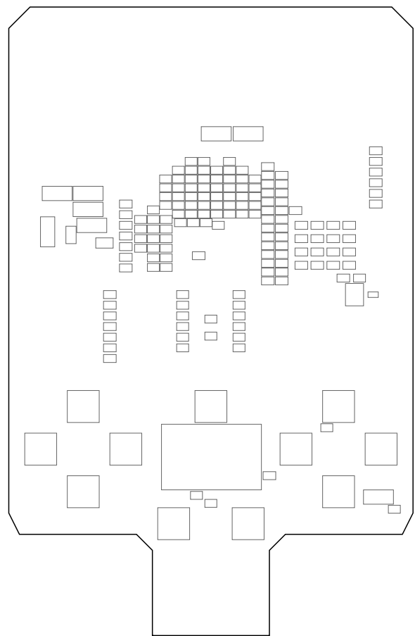
BOTTOM - source X/Y coordinates
