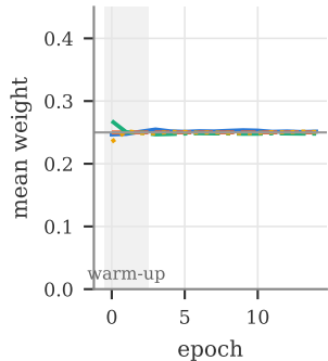
(d) T3 mean gate weight
