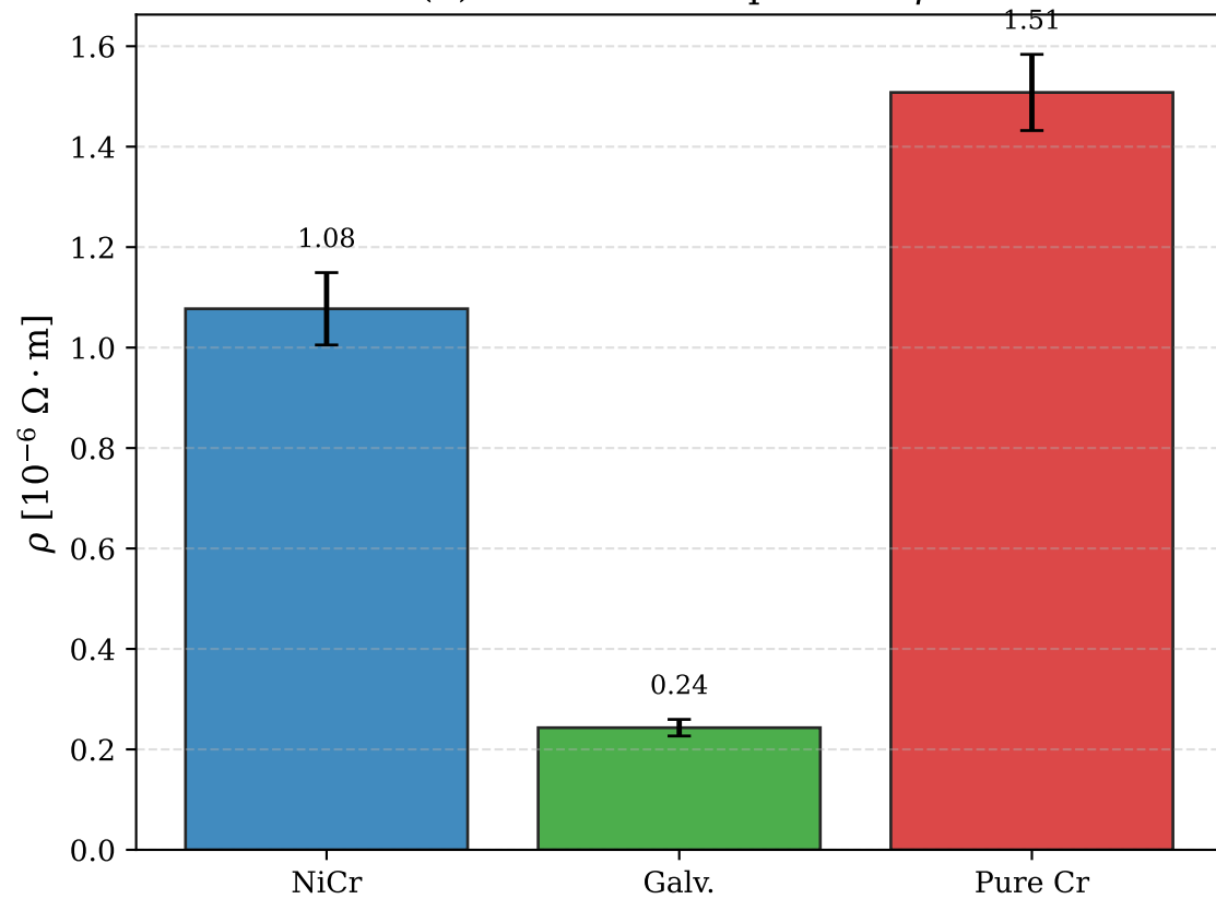
(d) Material Comparison: \rho
