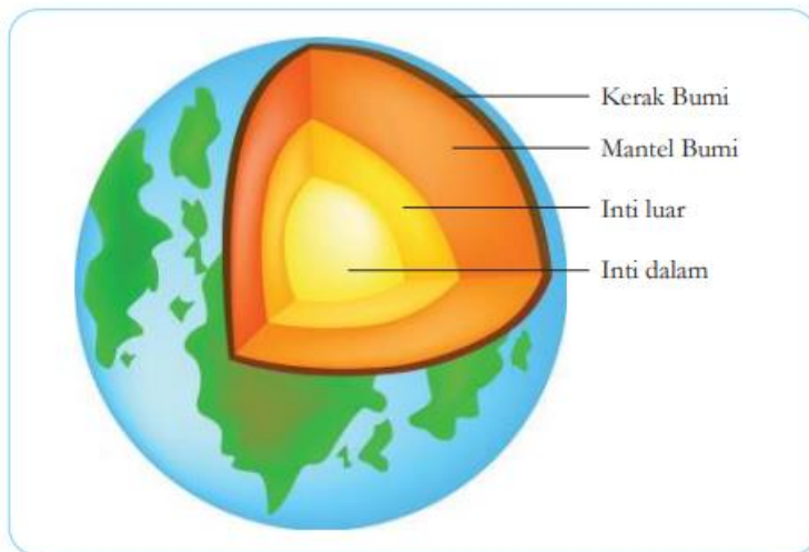
Gambar 2. Struktur bumi
