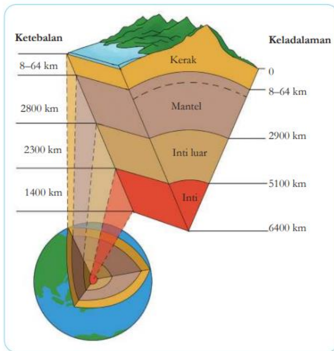
Gambar 4. Perbandingan ketebalan dan kedalaman setiap lapisan bumi.
