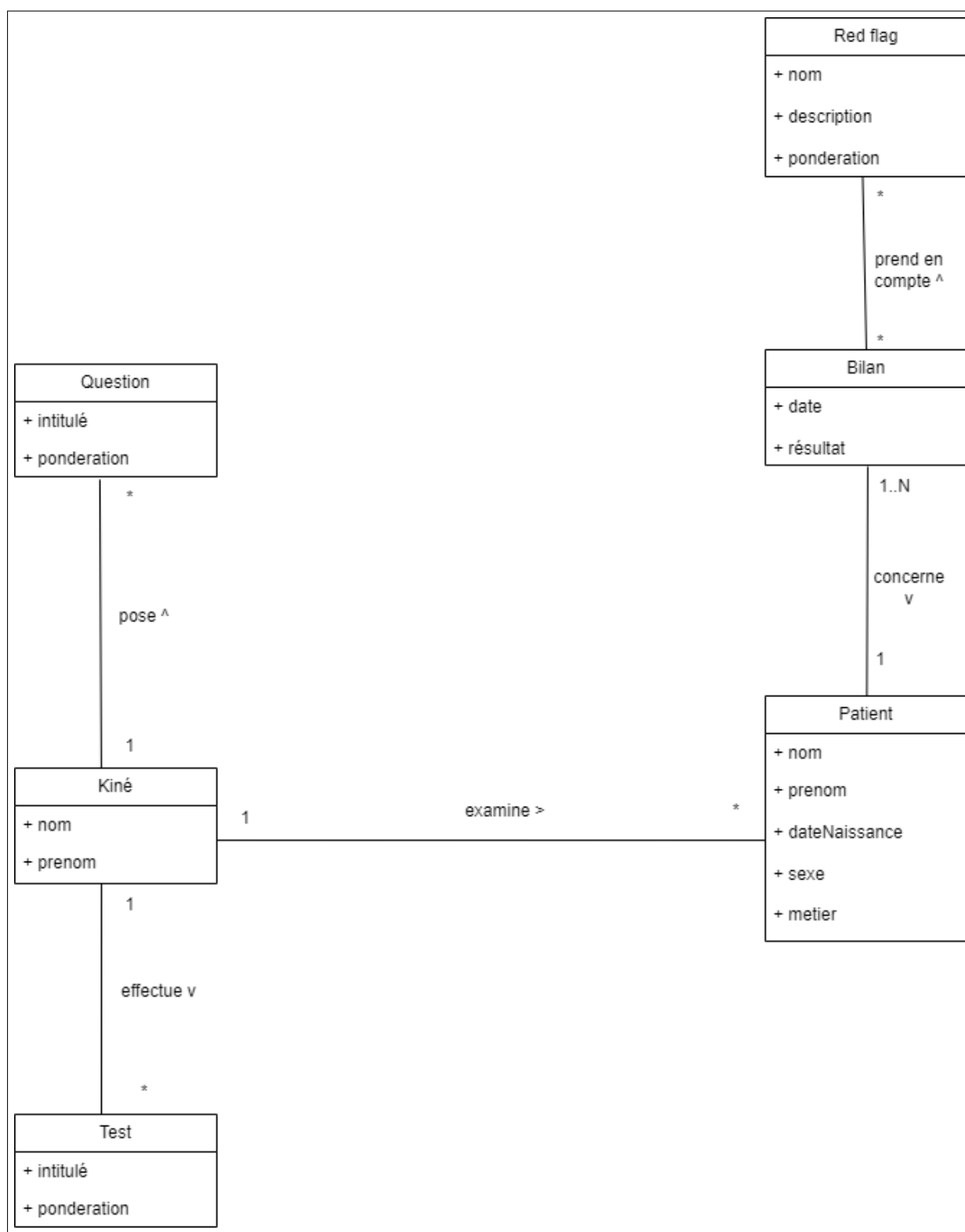
FIGURE 1.11 – Premier jet du diagramme de classe
