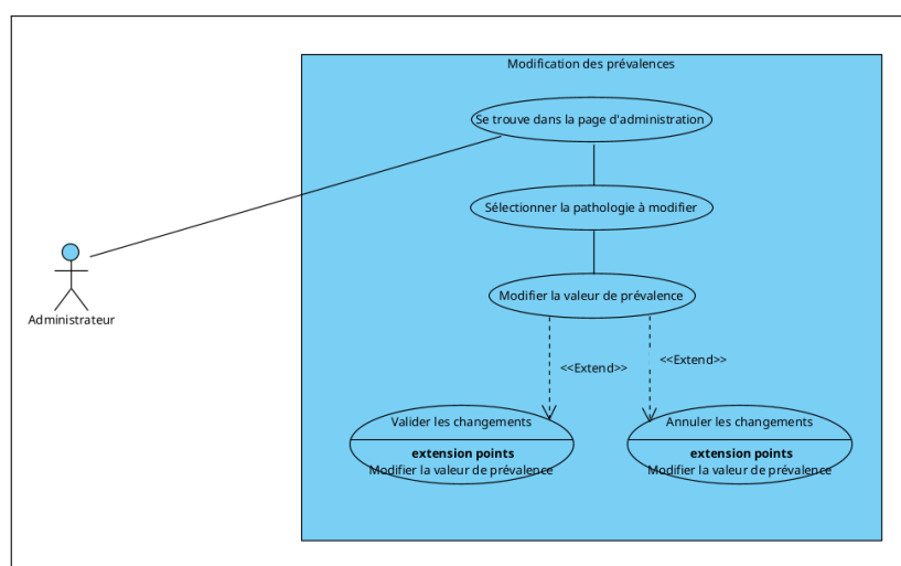
FIGURE 1.14 – Use case de modification des prévalences
