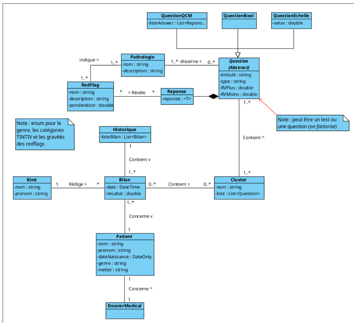
FIGURE 1.16 – Second jet du diagramme de classe
