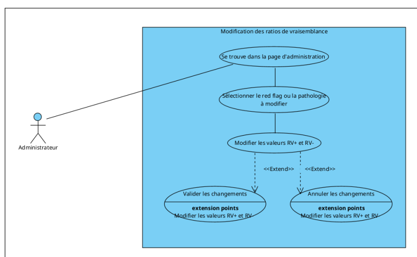
FIGURE 1.15 – Use case de modification des vraisemblances
