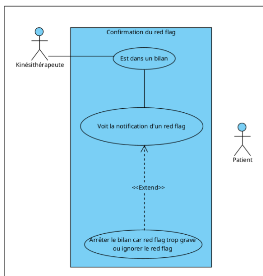
FIGURE 1.13 – Use case de l'apparition d'un red flag lors d'un bilan
