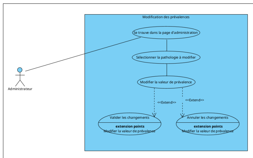
FIGURE 1.15 – Use case de modification des prévalences
