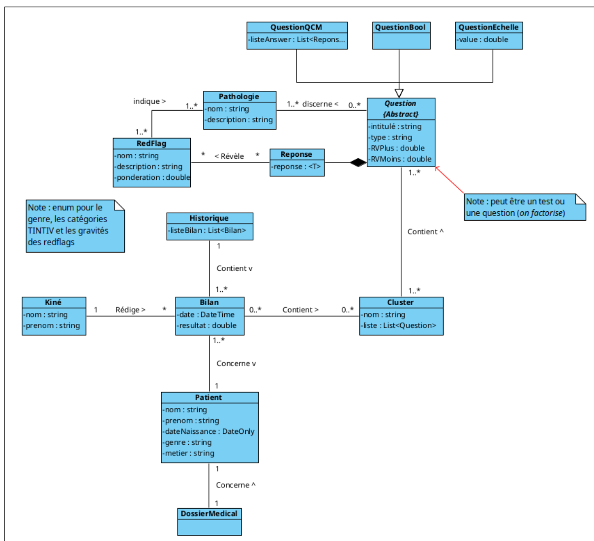
FIGURE 1.17 – Second jet du diagramme de classe
