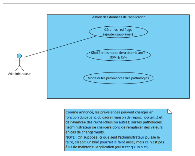
FIGURE 1.14 – Use case de l'administration de l'application
