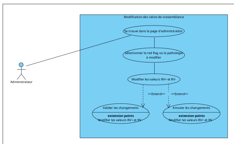
FIGURE 1.16 – Use case de modification des vraisemblances
