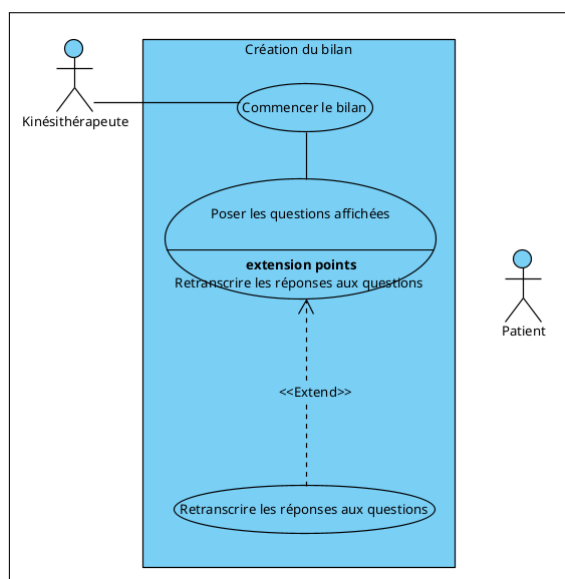
FIGURE 1.9 – Use case de la création du bilan
