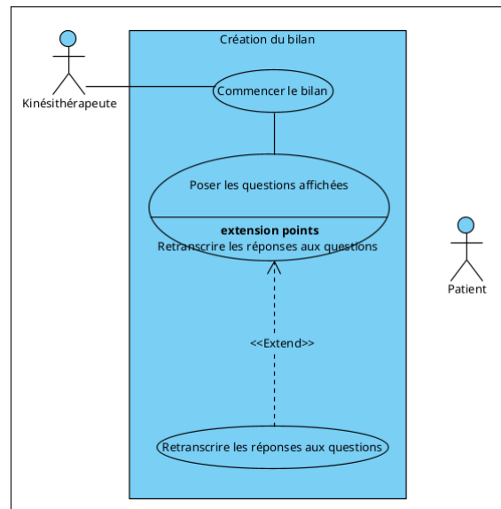
FIGURE 1.9 – Use case de la création du bilan
