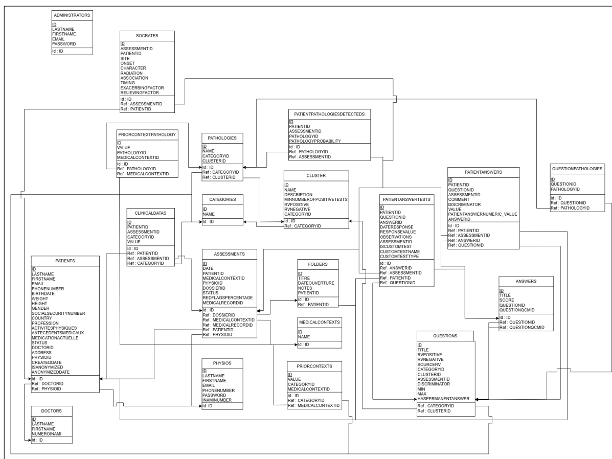
FIGURE 1.18 – Diagramme relationnel
