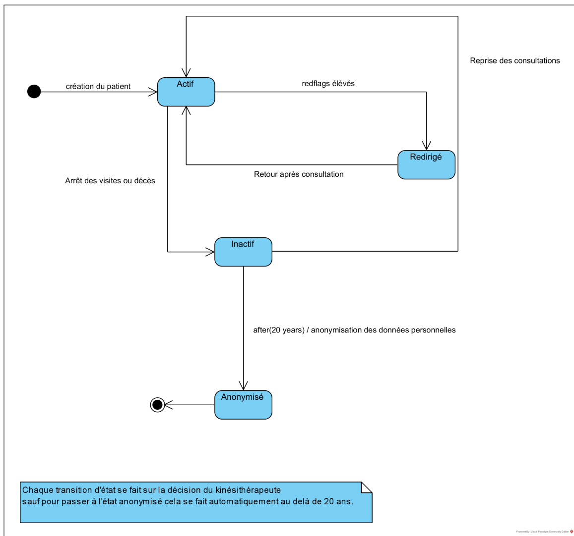
FIGURE 1.19 – Diagramme d'état pour le patient
