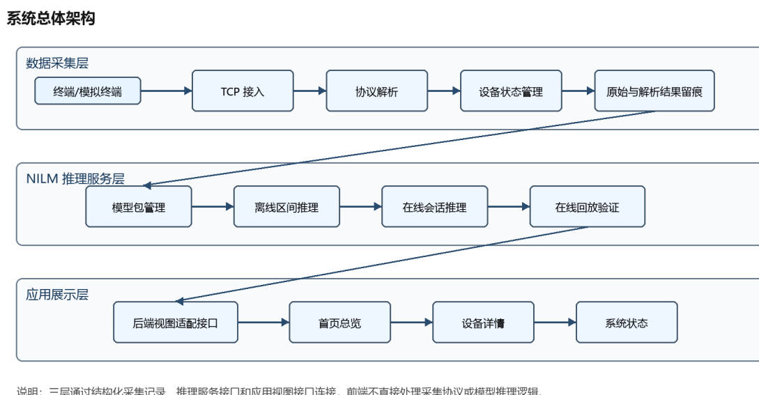
图 3-1 系统总体架构图
