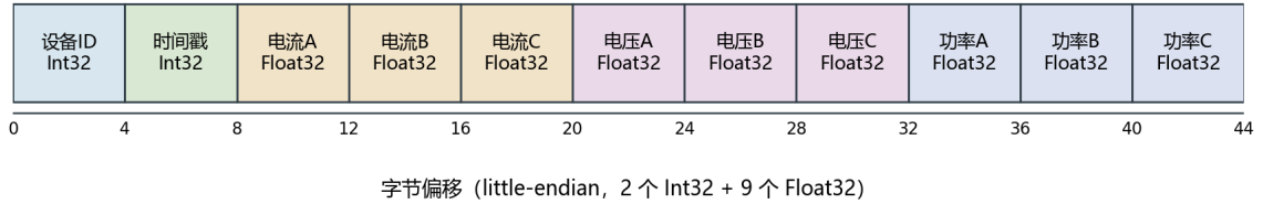
图 4-4 44 字节量测报文结构示意图
