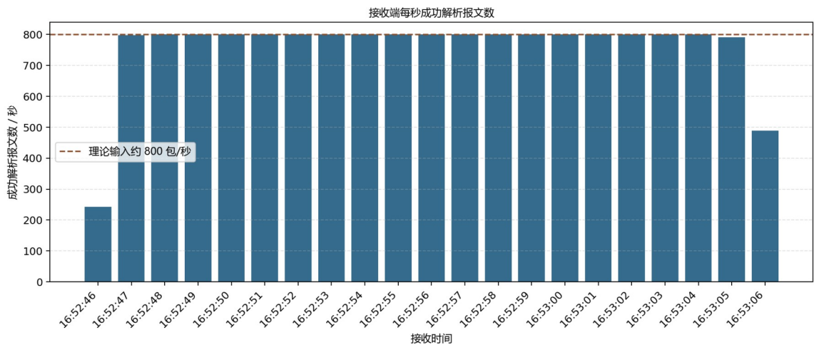
图 4-3 接收端每秒成功解析吞吐图
