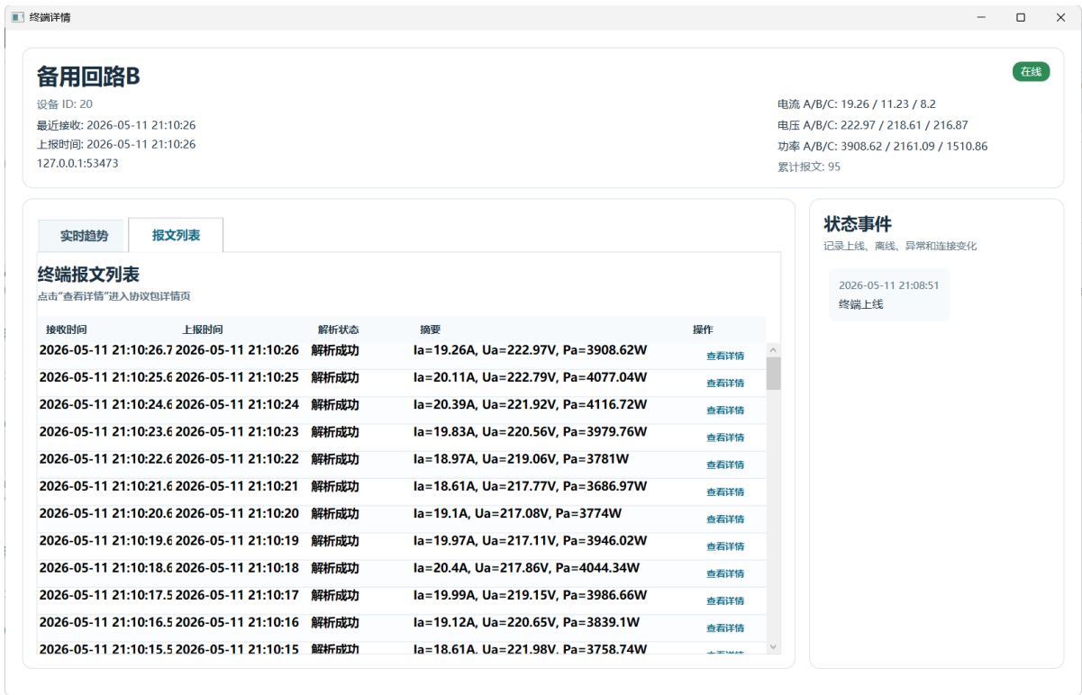
图 4-5 单终端报文列表展示
