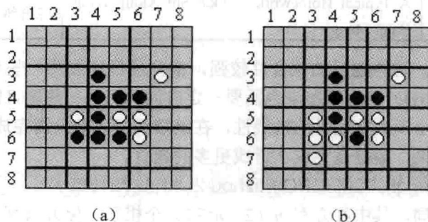
图 4-6 黑白棋
