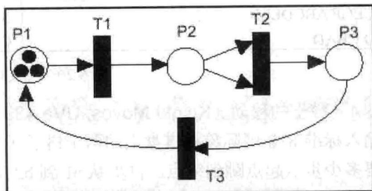
图 6-24 Petri 网模拟
