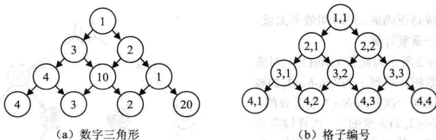
图 9-1 数字三角形问题
