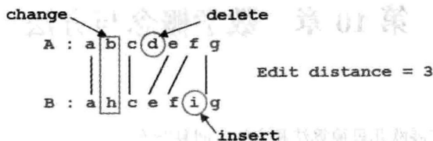
图 9-36 编辑距离
