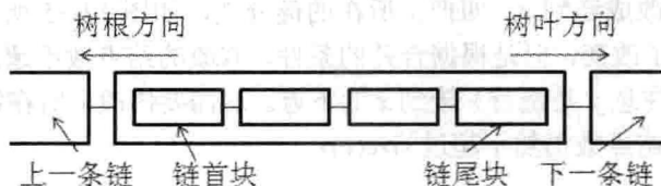
图 12-32 用块链表维护每条重路径
