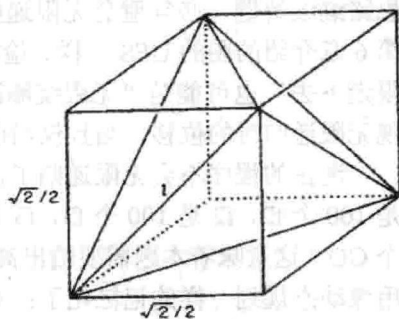
图 12-60 正四面体
