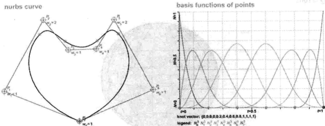
图 12-56 NURBS 曲线
