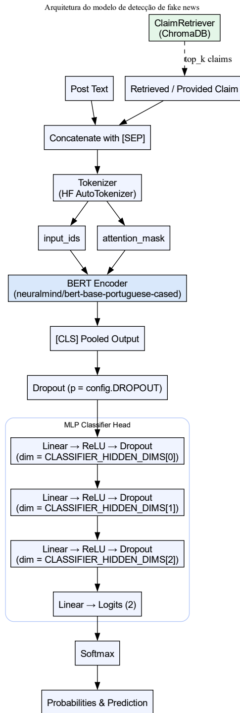
Figura 9: Arquitetura de ponta a ponta mostrando recuperação, processamento do cross-encoder e a head classifier MLP.
