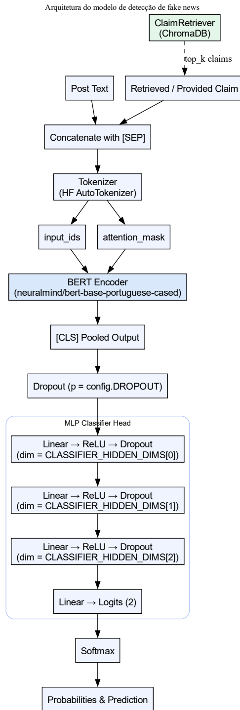
Figura 7: Arquitetura de ponta a ponta mostrando recuperação, processamento do cross-encoder e a head classifier MLP.
