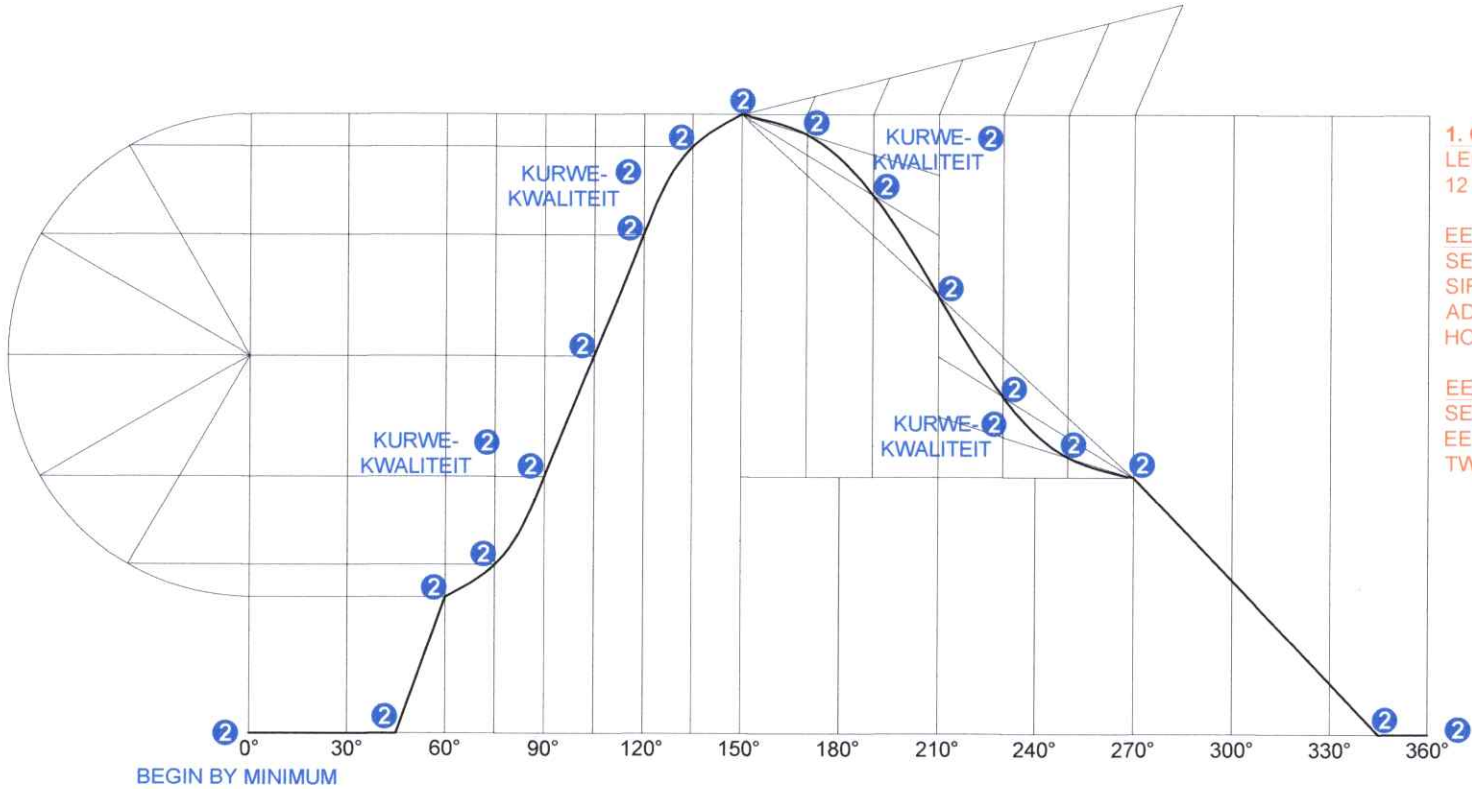
VERPLASINGSGRAFIEK ③ SKAAL 156 = 360° ③
