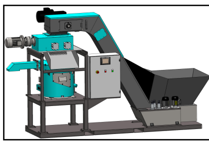
KOMBI-40 T TRITURATORE TR1 - SHREDDER TR1
