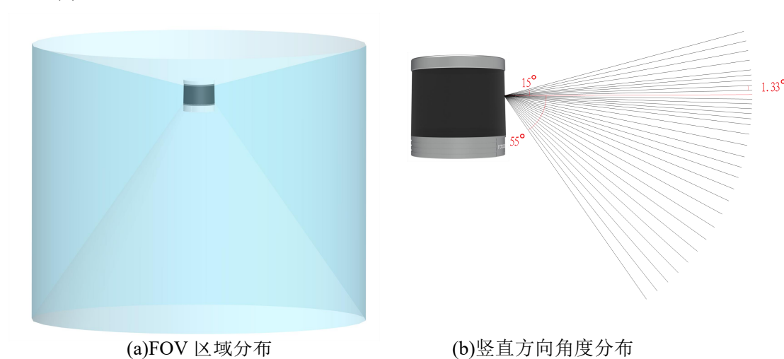
图 2 70° FOV 示意图
