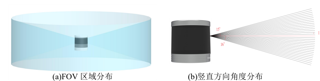
图 3 31° FOV 示意图
