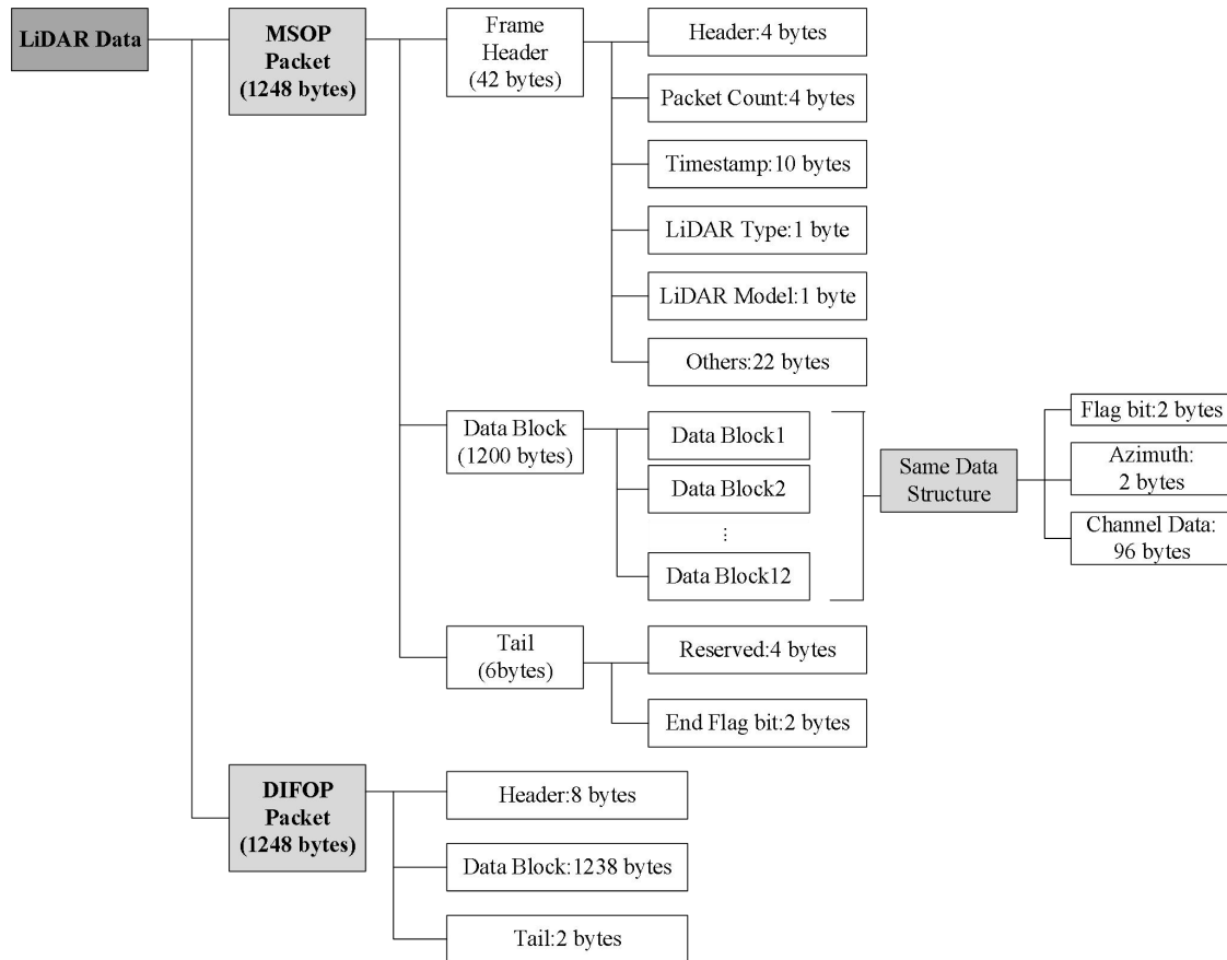
图 16 激光雷达数据结构示意图
