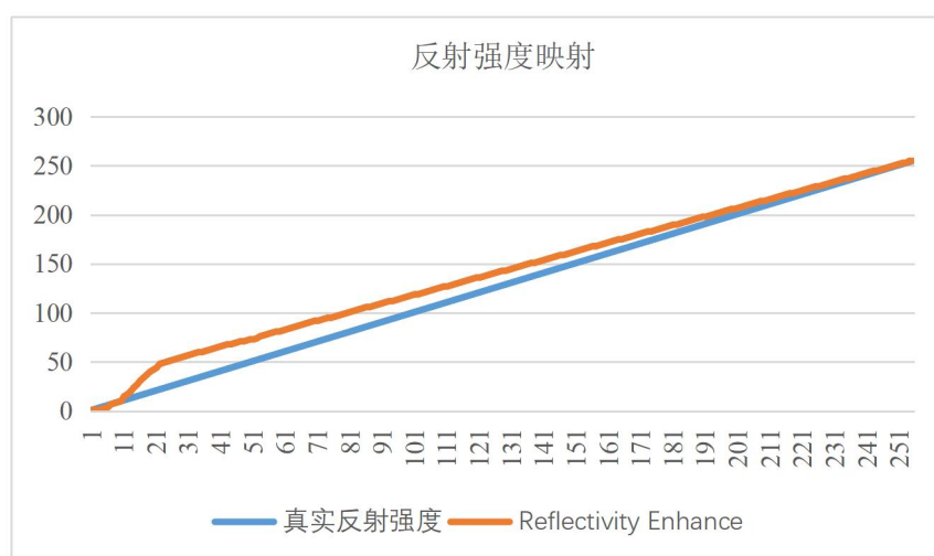
图 26 反射强度映射图
