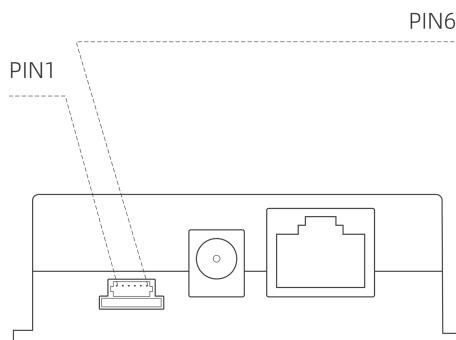
图 12 同步接口位置图
