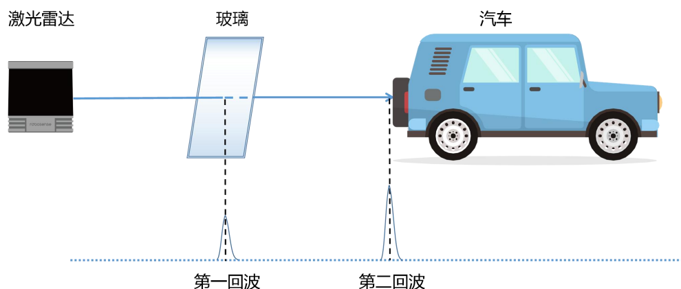
图 5 双回波检测
