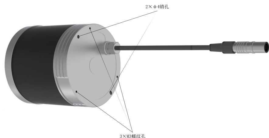
图 9 激光雷达底部定位销及螺丝示意图
