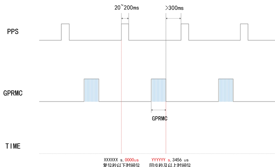
图 7 GPS 时间同步时序图
