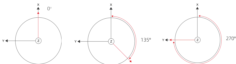
图 6 Helios 32 不同相位设定示意图
