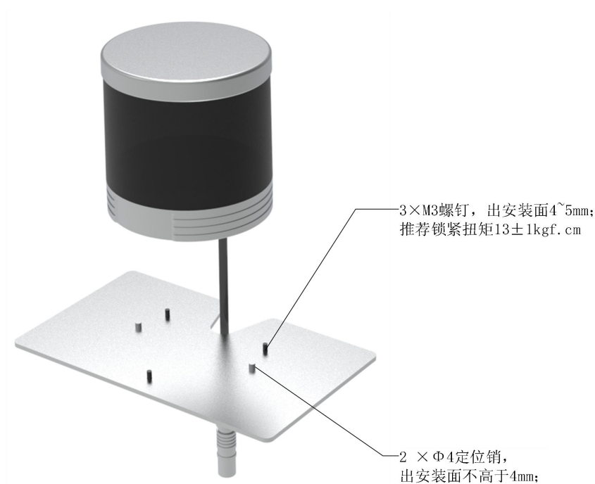
图8 激光雷达结构安装示意图
