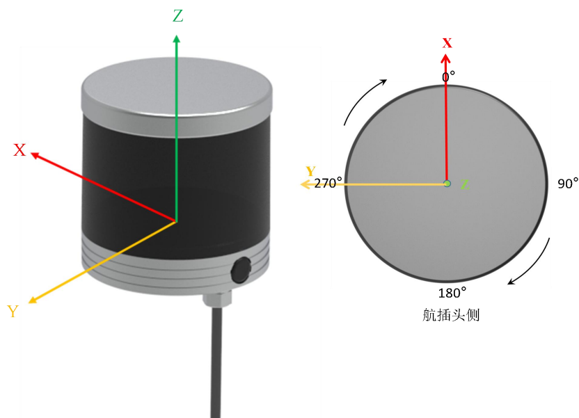
图 15 激光雷达坐标及旋转方向示意图
