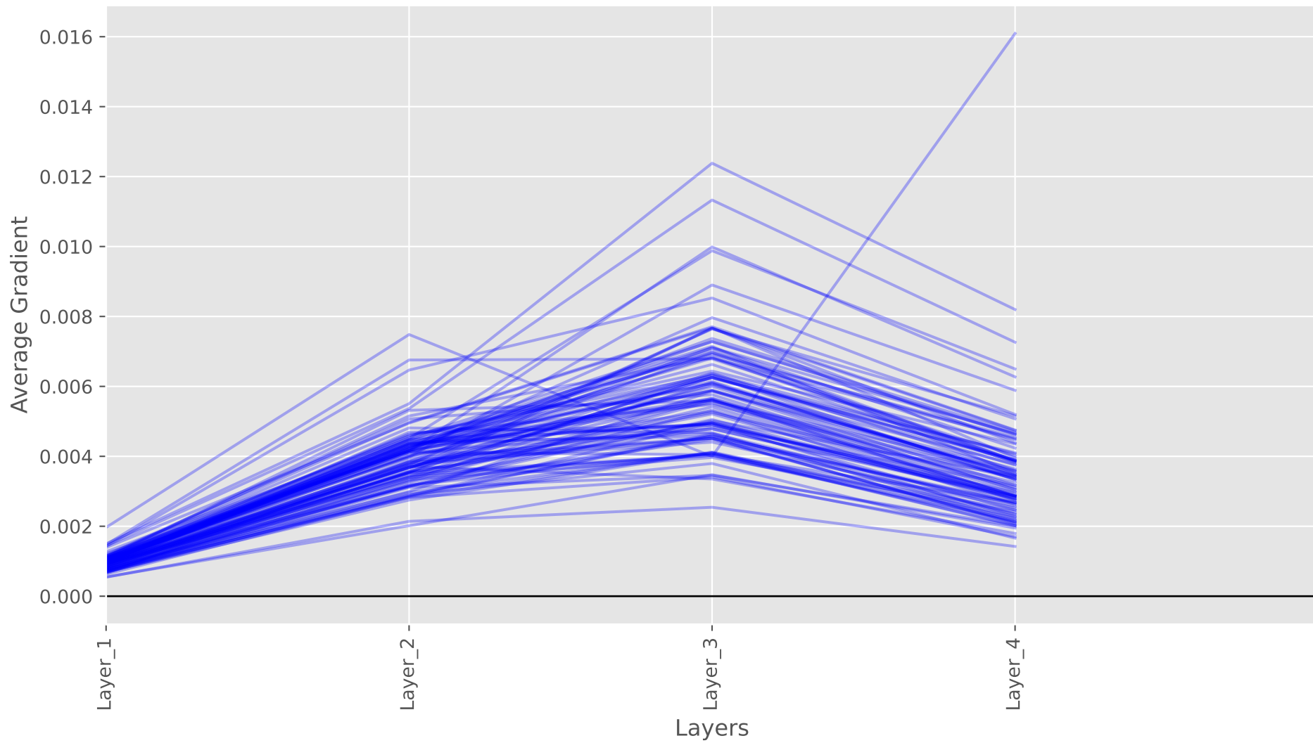
Gradient flow
