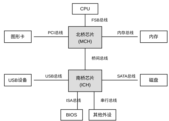
图6.2 南北桥结构示意图
