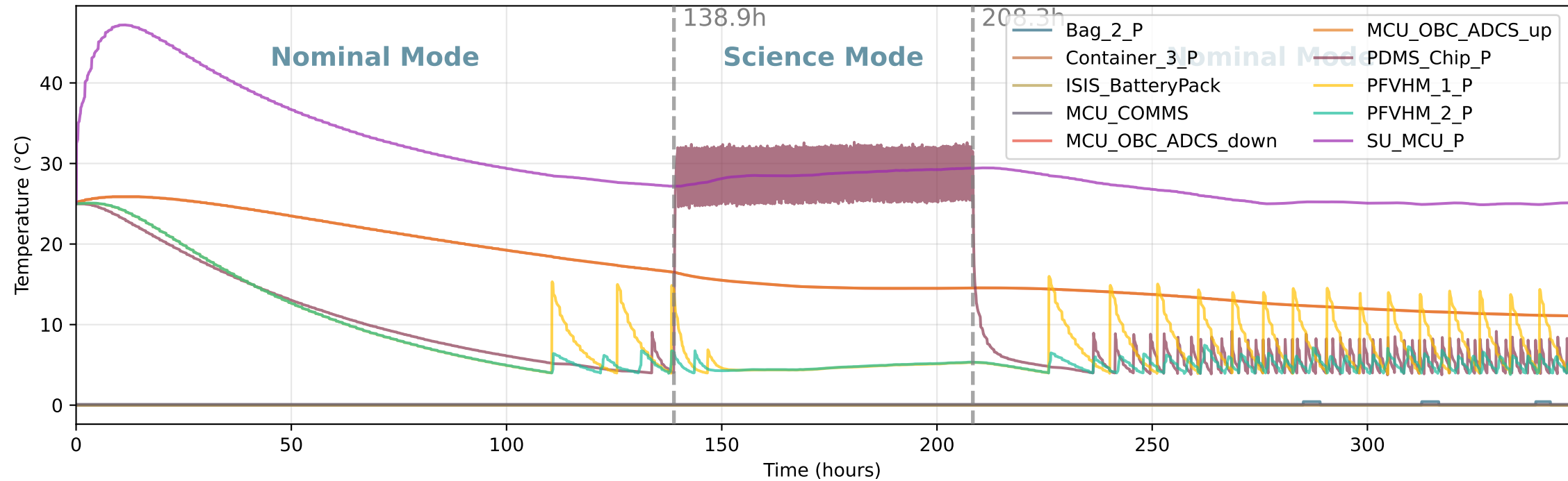
Acubesat_11_12_25 - Temperatures
