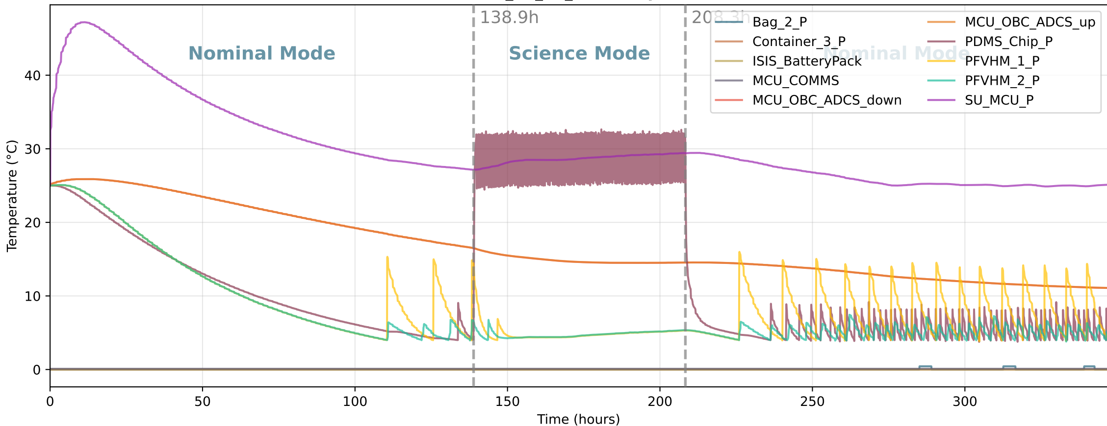
Acubesat_11_12_25 - Temperatures
