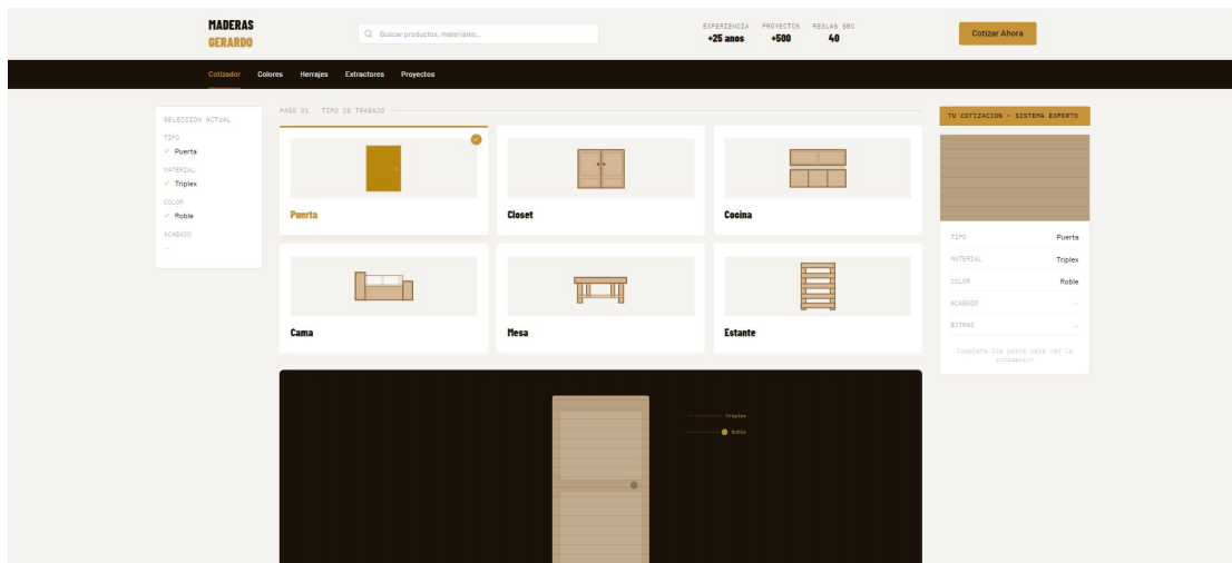
Figura 2. Cotizador con seleccion de tipo de mueble y panel del sistema experto.
