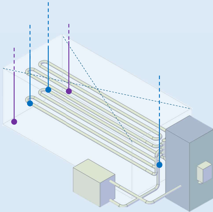
TC non gainés implantés dans le sable et sur les tubes
