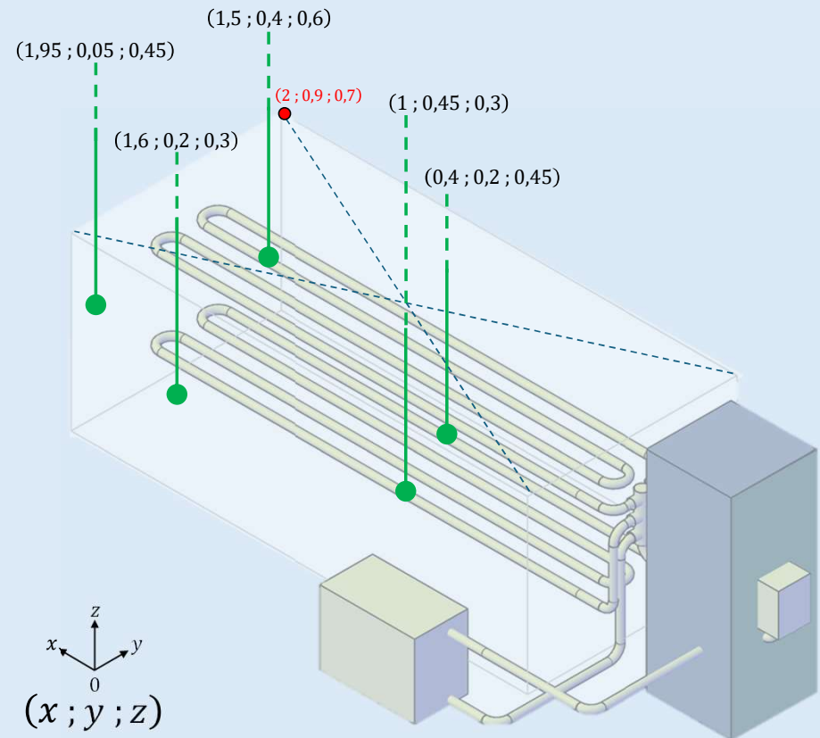
TC gainés inox implantés dans le sable
