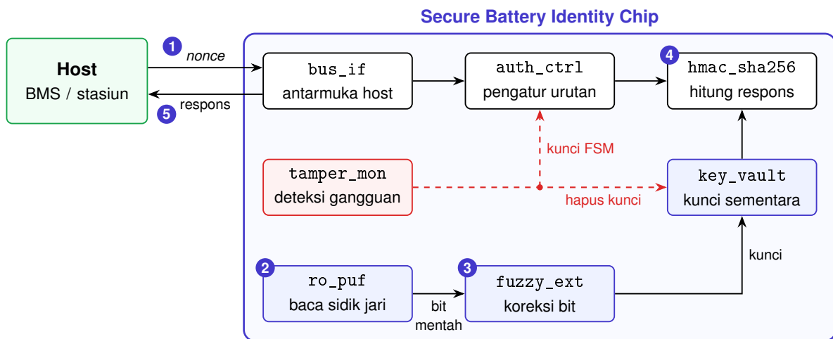
Gambar 2. Arsitektur chip. Nomor menunjukkan urutan satu autentikasi.
