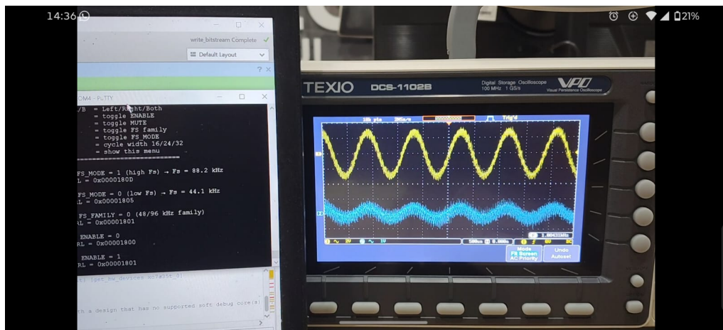
Gambar L.9. Hasil capture osiloskop: Enable=1 (enabled) - I2S transmitter aktif mengoutput audio
