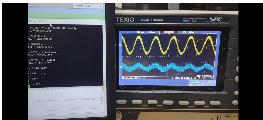
Gambar L.5. Hasil capture osiloskop: Audio tone 1 kHz - menunjukkan periodisitas sinyal I2S pada frekuensi 1 kHz
