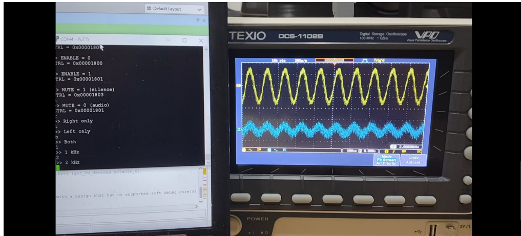
Gambar L.6. Hasil capture osiloskop: Audio tone 2 kHz - verifikasi laju sampling pada frekuensi 2 kHz
