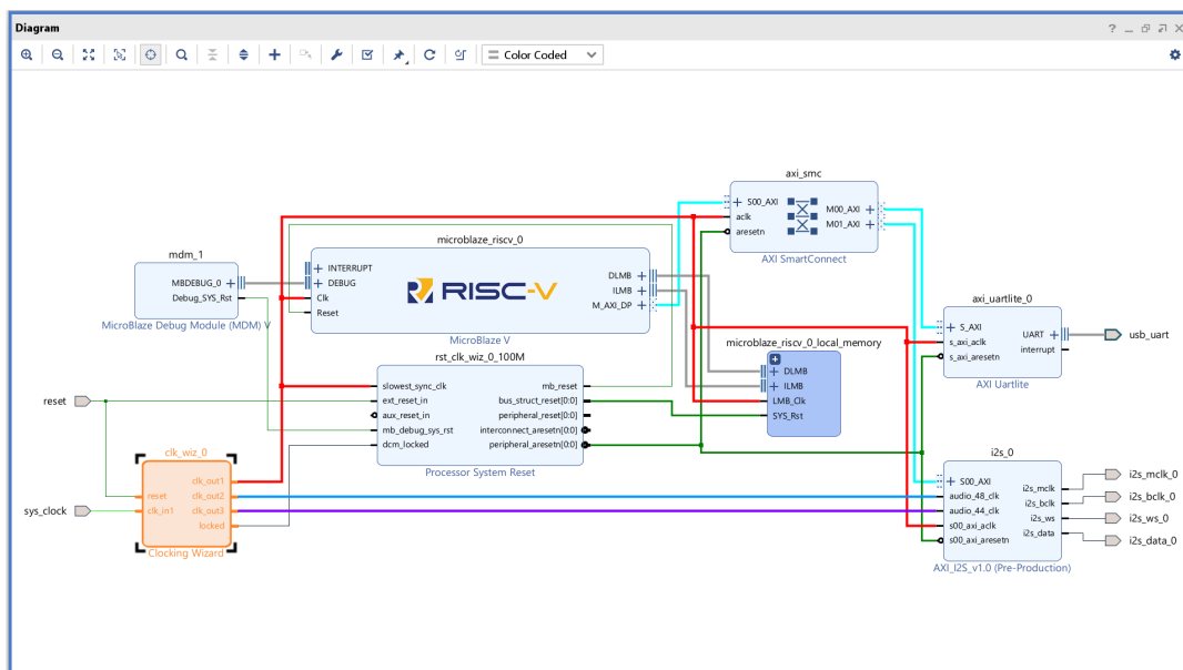
Gambar L.1. Diagram block warna-warni: arsitektur SoC beserta peripheral utama dan domain clock.
