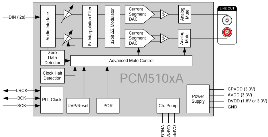
Gambar 4.7. Diagram blok fungsional PCM5102A dari dokumentasi Texas Instruments.
