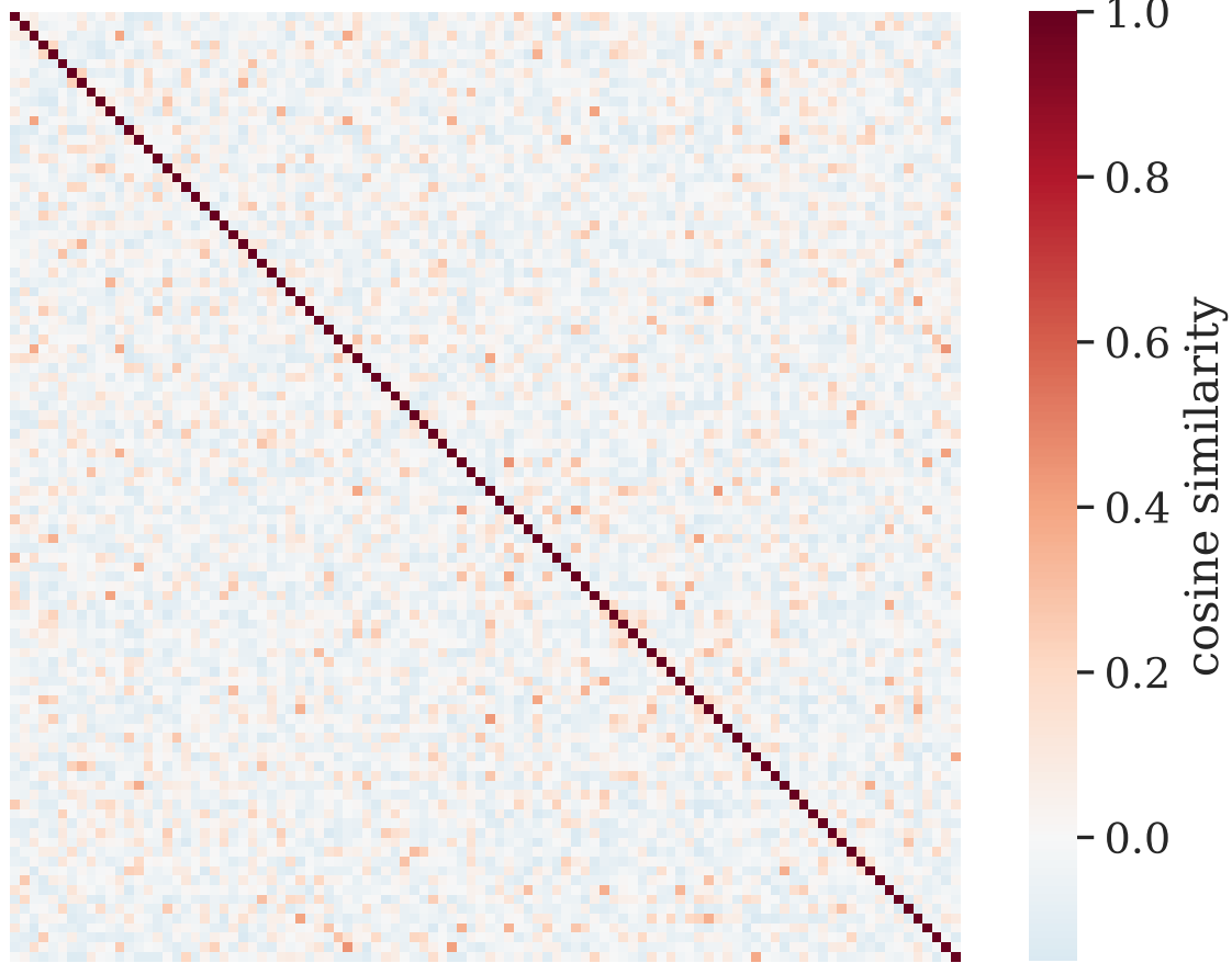
Actual Gram matrix
