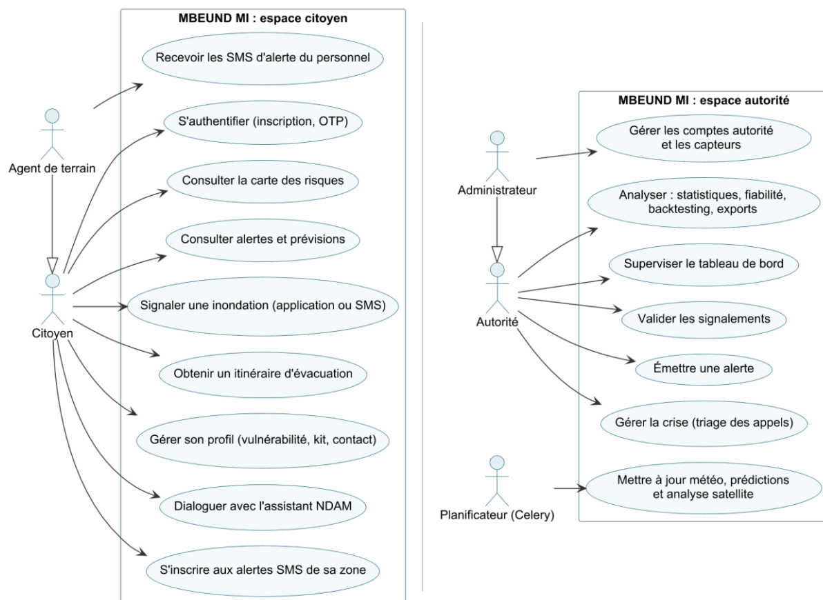
Figure 6 : Diagramme de cas d'utilisation de MBEUND MI
