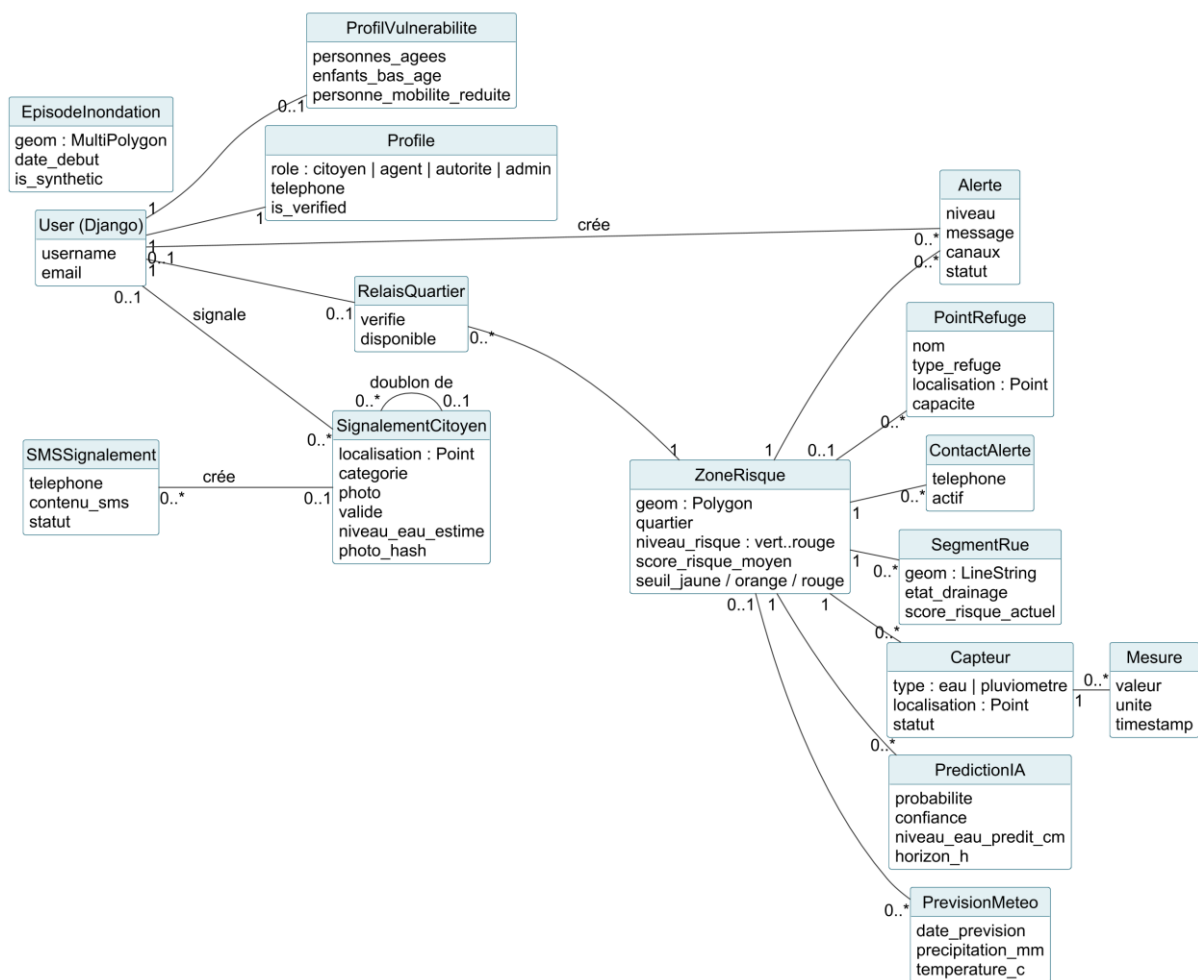
Figure 7 : Diagramme de classes simplifié de MBEUND MI
