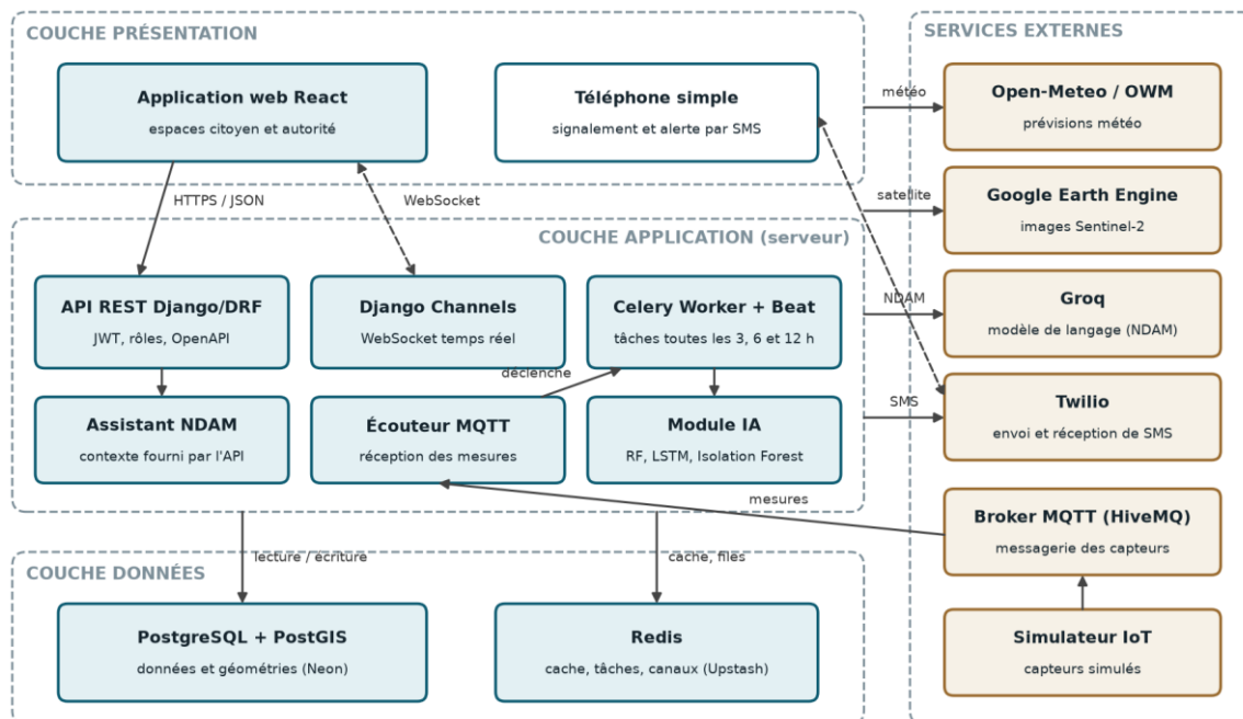
Figure 5 : Architecture logique de MBEUND MI
