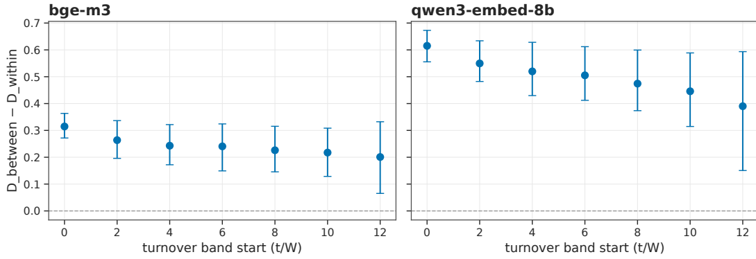
Рис. 4: Between-seed last-band gap против оборота в bge-m3 и qwen3-embed-8b на locked-панели этапа 5. Last-band CI исключают 0 сверху в обоих пространствах.
