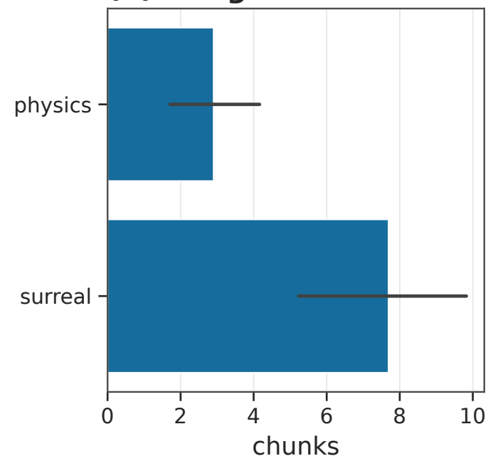
(d) integrated autocorrelation time
