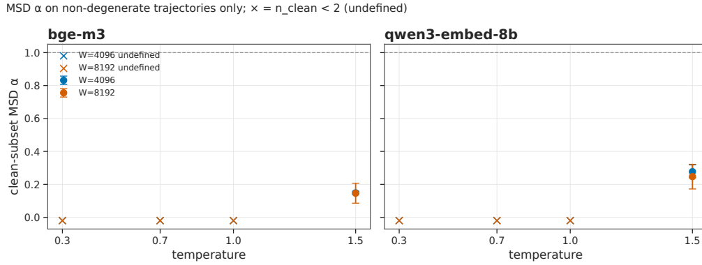
Рис. 3: Чистая MSD \alpha там, где определена (только не-looping ячейки). Отсутствующие точки при низком T — отсутствие H5.
