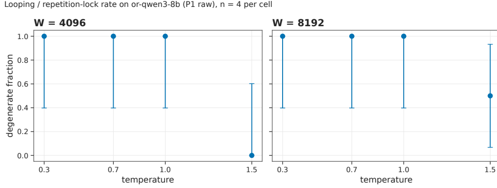
Рис. 2: Частота looping против температуры на двух окнах, 95% CI Clopper–Pearson, n=4 . Ячейка T=1.5 , W=4096 — существование не-looping режима на этой модели, а не время перемешивания.
