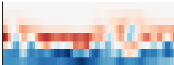
Gradient magnitude
