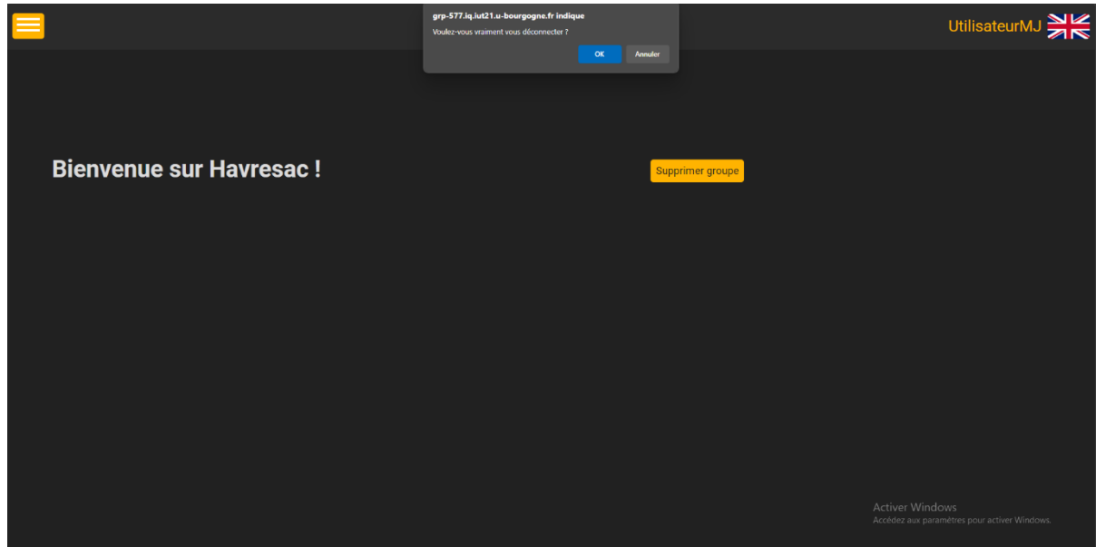
Figure 5 Déconnexion
