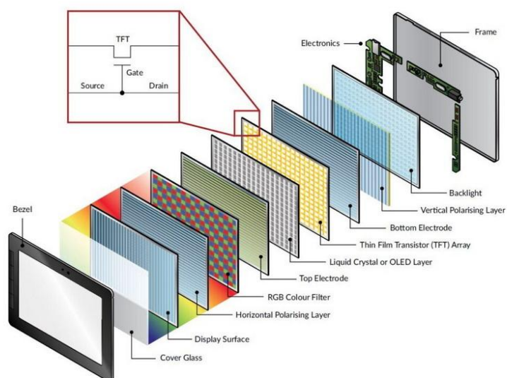
Obrázek č. 14 LCD / Jednotlivé vrstvy displeje
