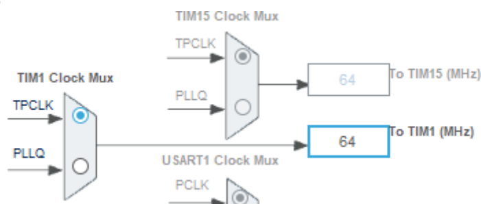
Obrázek č. 5 TIM1 / Nastavení hodin
