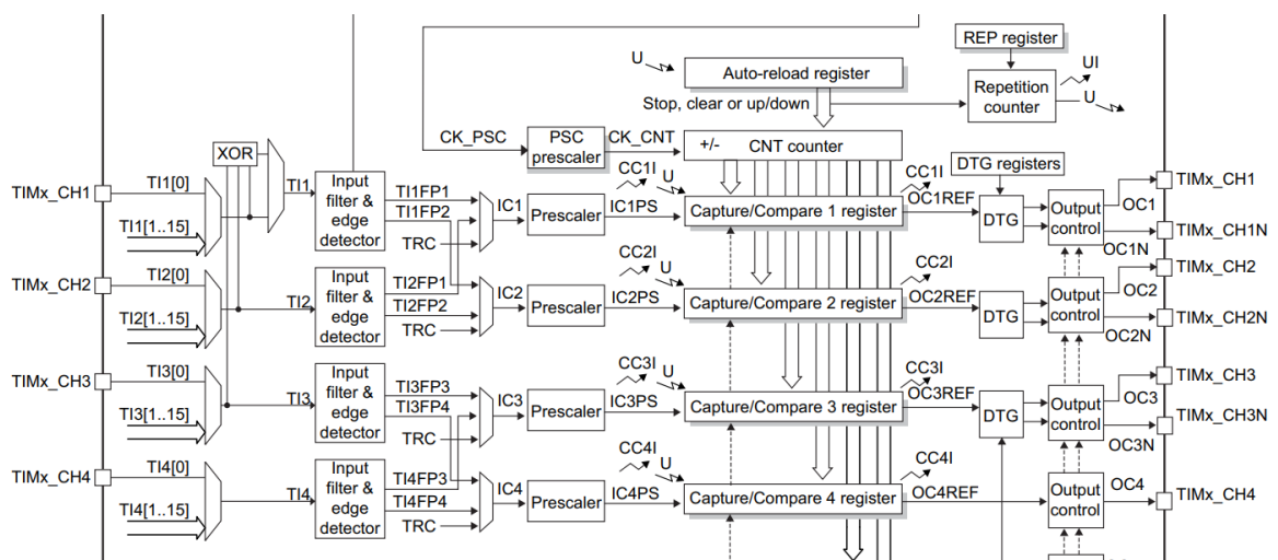
Obrázek č. 4 TIM1 | Blokové schéma
