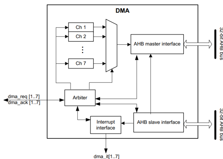
Obrázek č. 7 DMA / Blokový diagram DMA kontroléru
