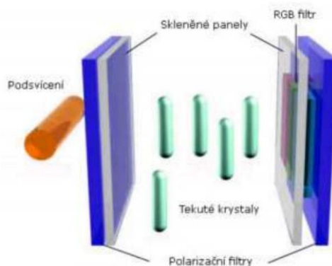
Obrázek č. 13 LCD / Konstrukce barevného LCD
