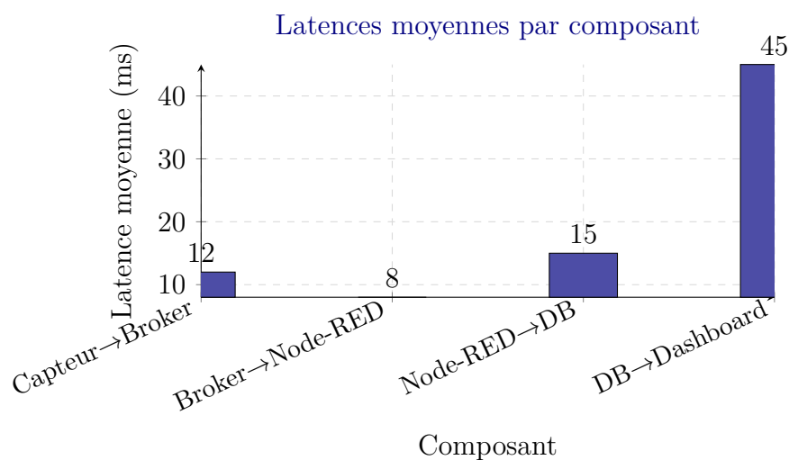
FIG. 4.2 : Latences moyennes mesurées par composant
