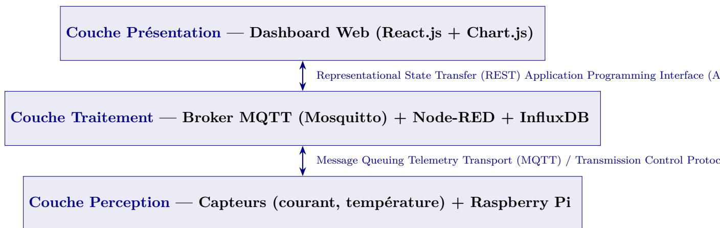
FIG. 2.1 : Architecture trois-tiers de la plateforme IoT
