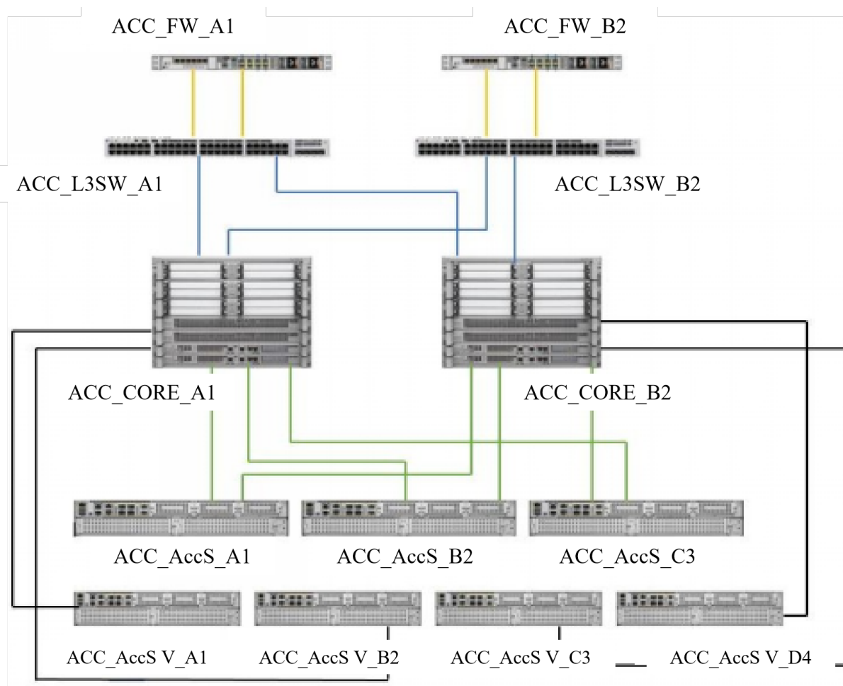
FIG. 2.2 : Architecture au sein du CRCSNA Casablanca.
